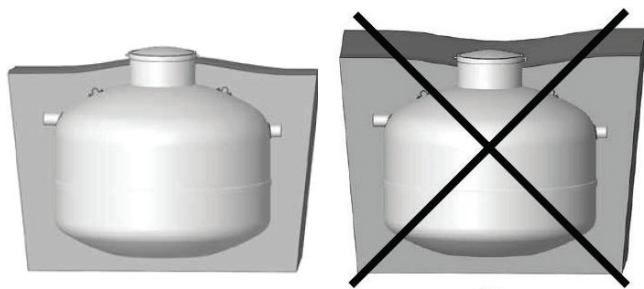
Figur 1: Riktig avrenning.
