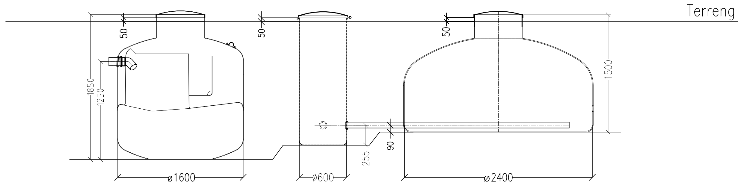
2m3 Slamavskiller
